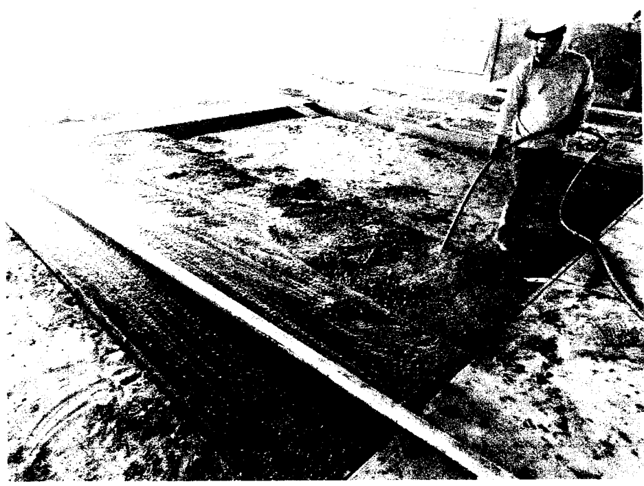
IMAGEN 07 - LLENADO DE PISO, UTILIZANDO VIBRADOR PARA EVITAR CANGREJERAS
